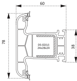
PRVNEC03B Orta Kayıt Profili Mullion Profile
