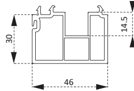
PRTS87 Kasa Altı Montaj Prof ili Frame Under Montage Profile
