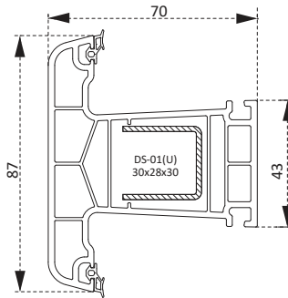
PDR0360BY Orta Kayıt Profili Mullion Profile
