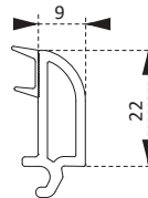
PSC9660BY 40 mm Cam Çıtası 40 mm Glazing Bead
