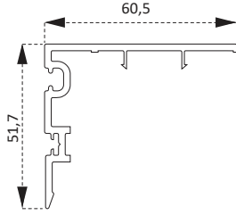
PSY3860BY Sürme Kanat Adaptörü Sliding Sash Adapter
