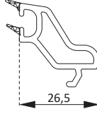
PR7120BY 24 mm Dekoratif Cam Çıtası 24 mm Decorative Glazing Bead
