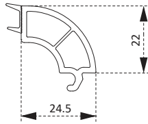
PSC1960BY 24 mm Cam Çıtası 24 mm Glazing Bead
