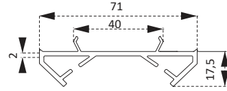
PDR2760BY Köşe Dönüş Adaptörü Corner Adapter
