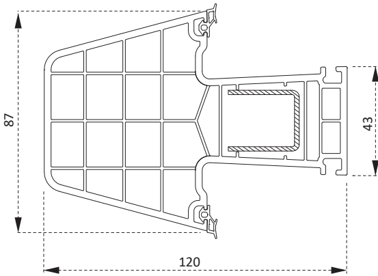
PRHL03 Orta Kayıt Profili Mullion Profile
