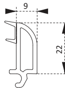
PSC9660BY 40 mm Cam Çıtası 40 mm Glazing Bead
