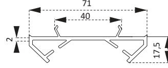
PDR2760BY Köşe Dönüş Adaptörü Corner Adapter
