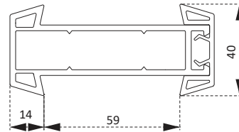
PEX2560BY Geniş Bağ Profili Wide Band Profile
