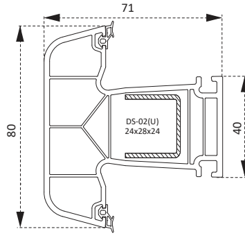
PV70360BY Orta Kayıt Profili Mullion Profile
