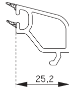
PR7119BY 24 mm Cam Çıtası 24 mm Glazing Bead
