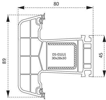
PGR0360BY Orta Kayıt Profili Mullion Profile
