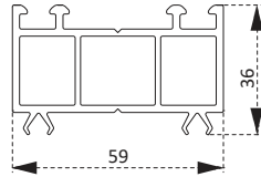
PEX3760BY Kasa Yükseltme Profili Frame Joint Profile
