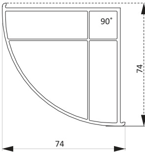
PDR3060BY 90° Köşe Dönüş Adaptörü 90° Corner Angle Adapter
