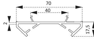
PDR2760BY Köşe Dönüş Adaptörü Corner Adapter
