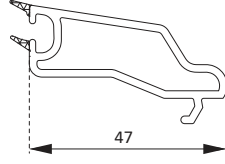
PR7114BY Tek Cam Çıtası Single Glazing Bead
