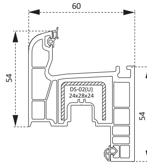
PRVNEC02B Kanat Profili Sash Profile
