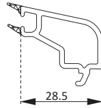
PR7117BY 20 mm Cam Çıtası 20 mm Glazing Bead
