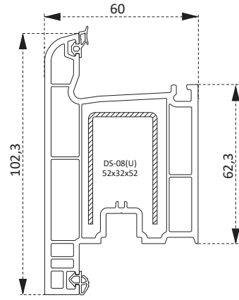
PVN0560BY Dış Açılım Kapı Profili Outside Opening Door Profile
