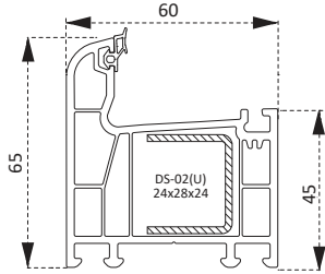
PRVNEC01B Kasa Profili Frame Profile
