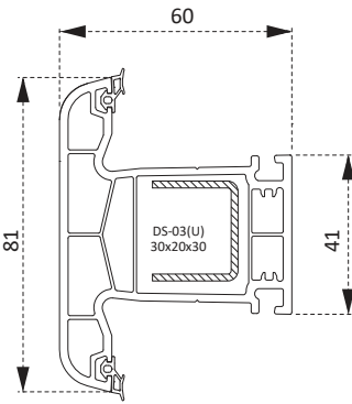
PVN0360BY Orta Kayıt Profili Mullion Profile
