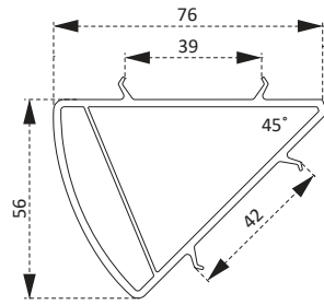
PDR2960BY 45° Köşe Dönüş Adaptörü 45° Corner Angle Adapter
