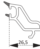
PDR2060BY 24 mm Dekoratif Cam Çıtası 24mm Decorative Glazing Bead
