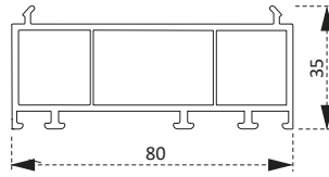
PSC3760BY.0001 Kasa Yükseltme Profili Frame Joint Profile
