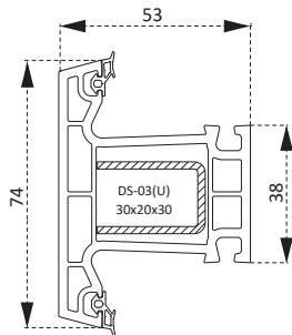
PFS0360BY Orta Kayıt Profili Mullion Profile
