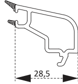
PDR1760BY 20 mm Cam Çıtası 20 mm Glazing Bead
