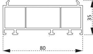
PSC3760BY.0001 Kasa Yükseltme Profili Frame Joint Profile
