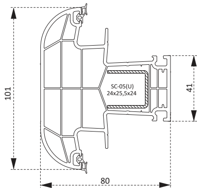
PSC0360BY Orta Kayıt Profili Mullion Profile
