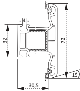
PS60360BY Orta Kayıt Prof Mullion Profile
