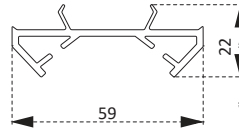
PEX2760BY Köşe Dönüş Adaptörü Corner Adapter
